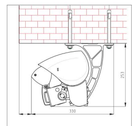
Deckenmontage mit Variovolant (Maße in mm)
