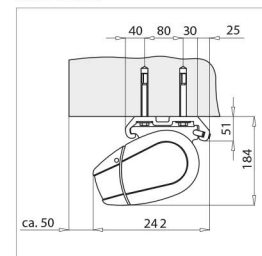
Deckenmontage (Maße in mm)
